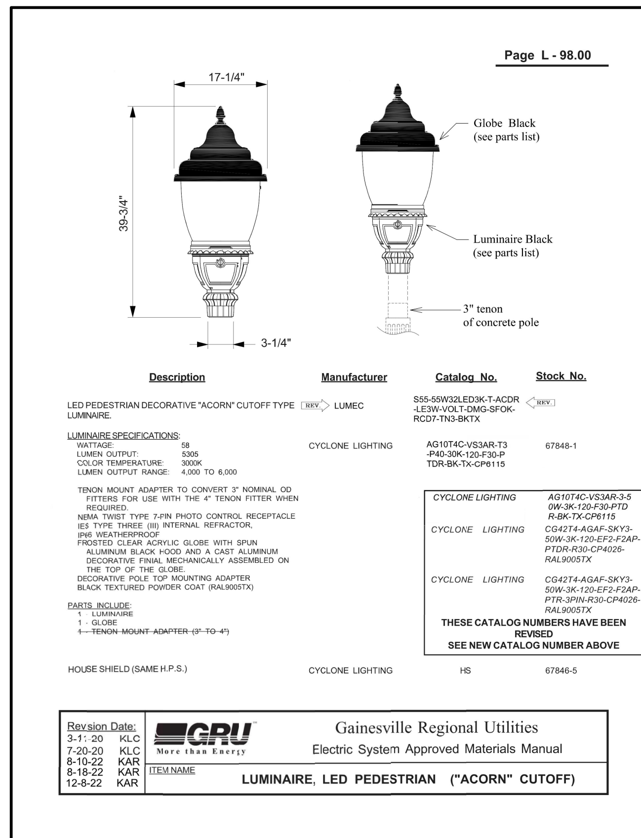
TYPE B LUMINAIRE
